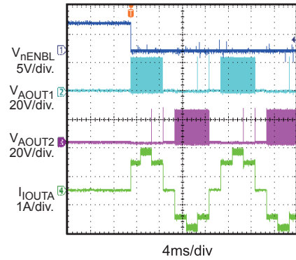
Enable-Half Step
