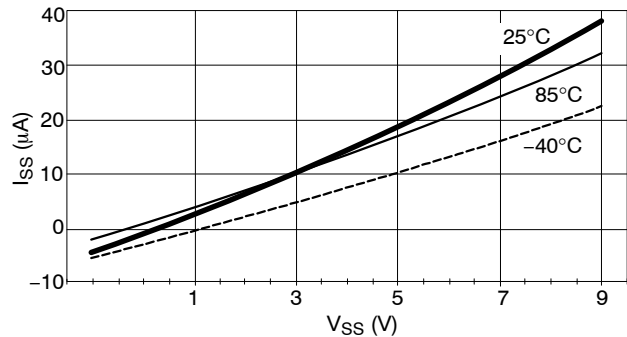
Figure 20. I_{SS} vs. V_{SS}
