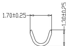
SEC:B-B
