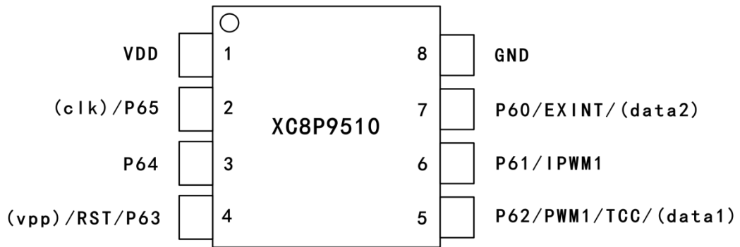
XC8P9510-8PIN 脚位图
