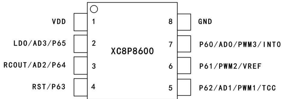
XC8P8600-8PIN 脚位图
