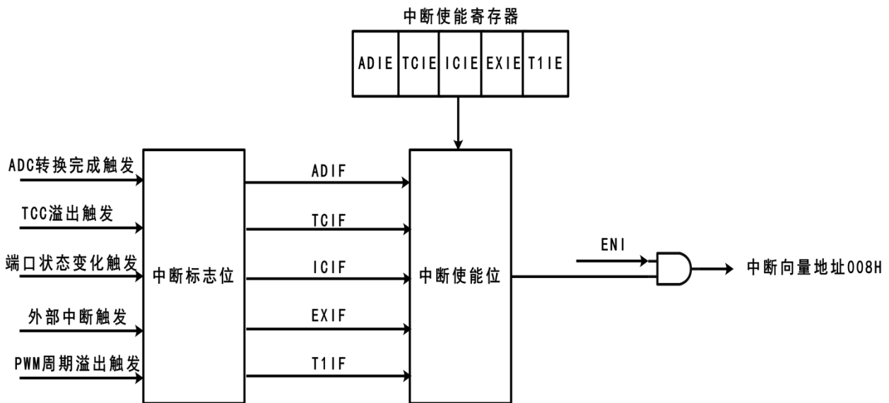
中断原理示意图
