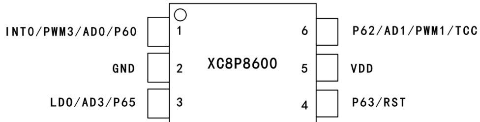
XC8P8600-6PIN 脚位图
