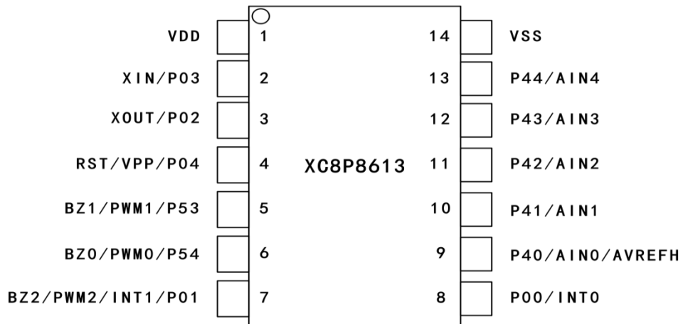
XC8P8613-14PIN 脚位图
