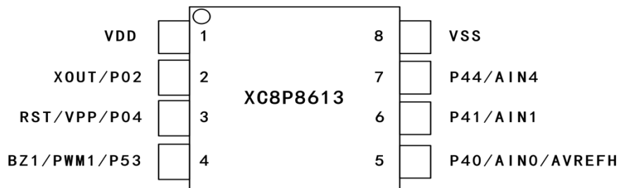
XC8P8613-8PIN 脚位图
