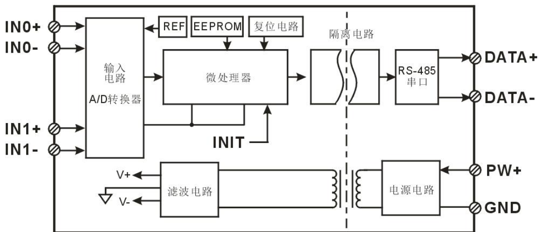
图2 YL20 模块内部框图
