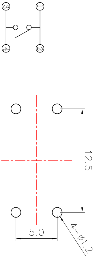
电器原理图
