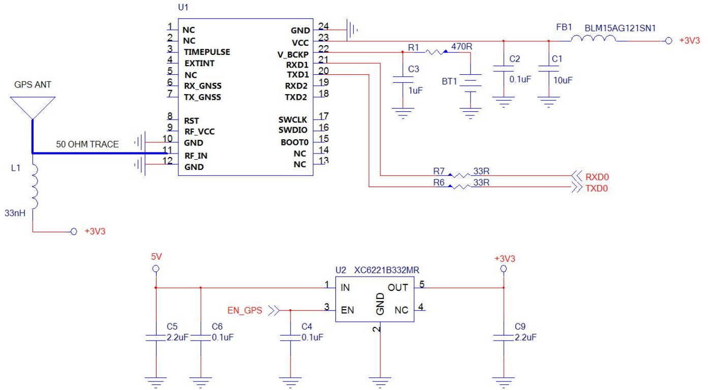
图 5: SKG123N 参考电路//Reference circuit
