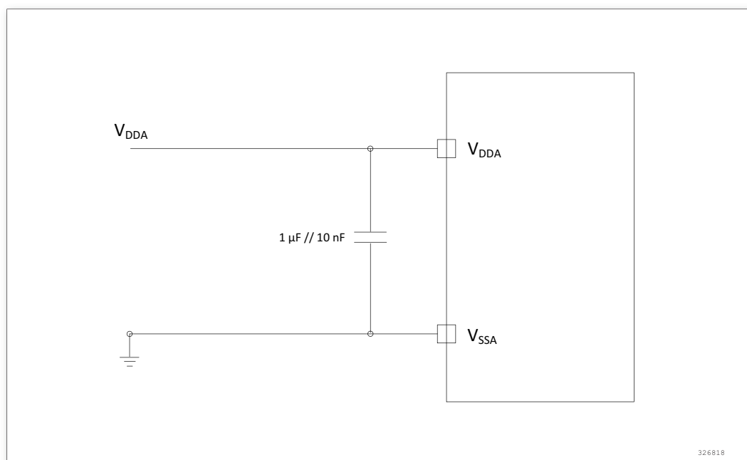
图 22. 供电电源和参考电源去耦线路
