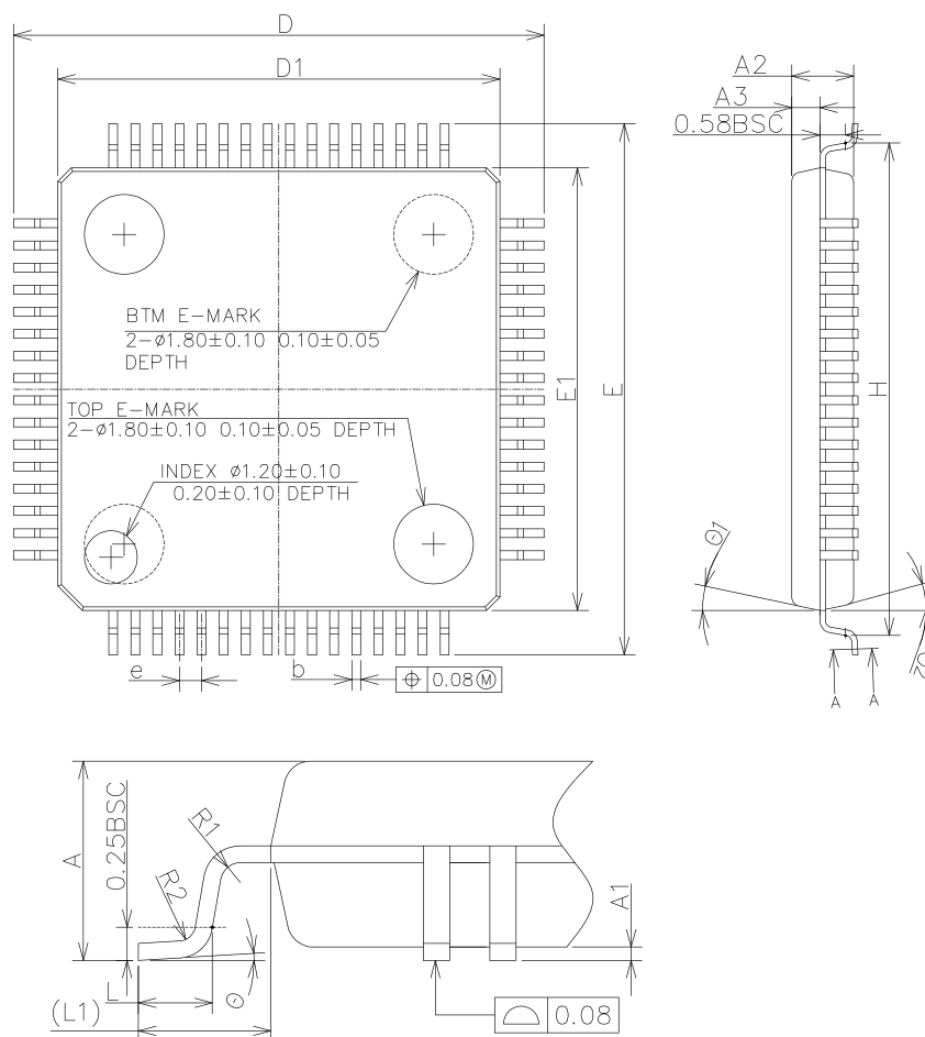
图 23. LQFP64, 64 脚低剖面方形扁平封装图
