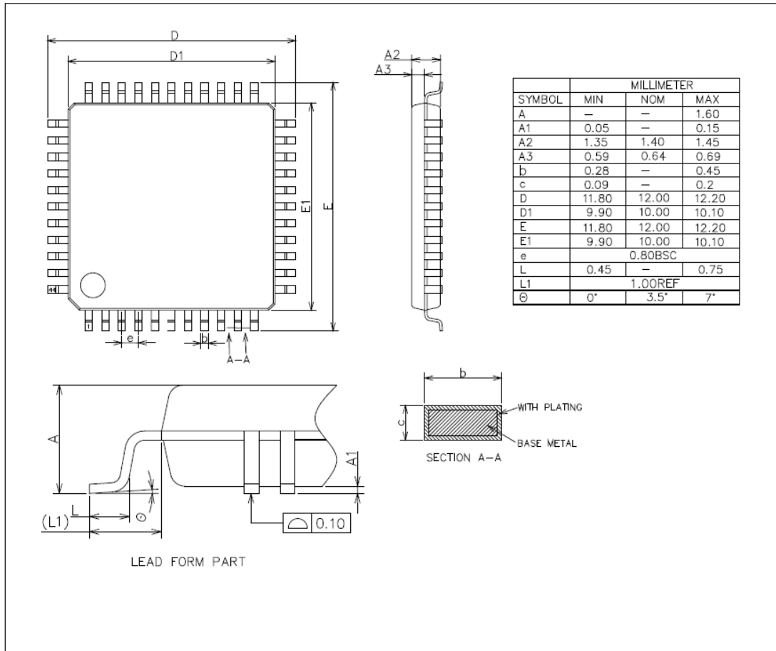
图 5 LQFP44 封装图
