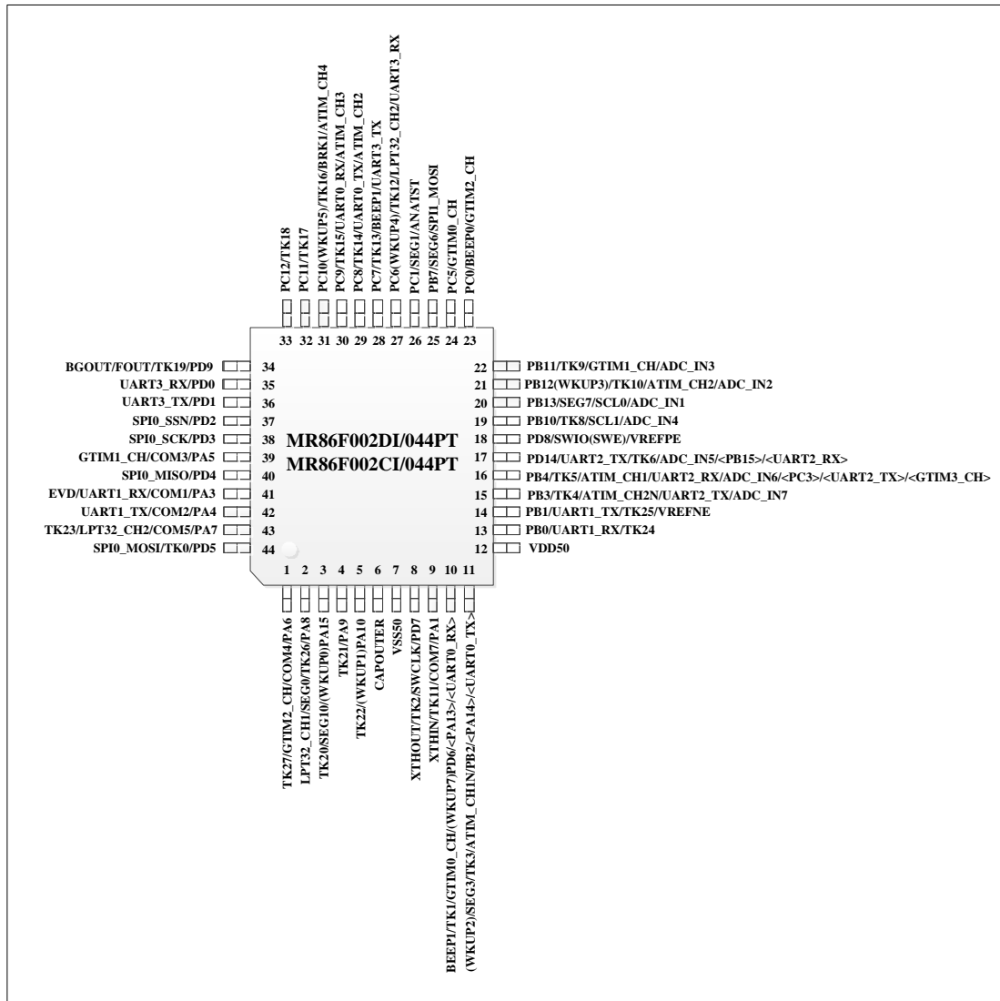
图 2 MR86F002 管脚分配图 (LQFP44)
