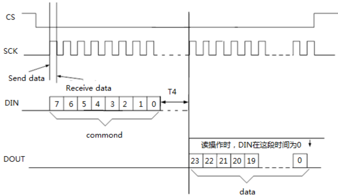
图3-3-1 读操作时序
