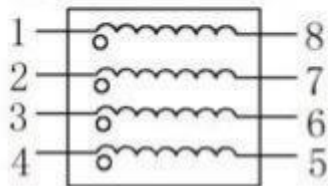
等效原理图
