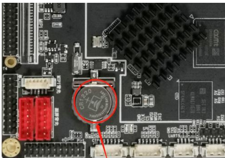
RTC电池座子
