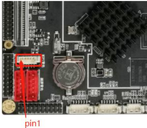
MIPI 背光接口
