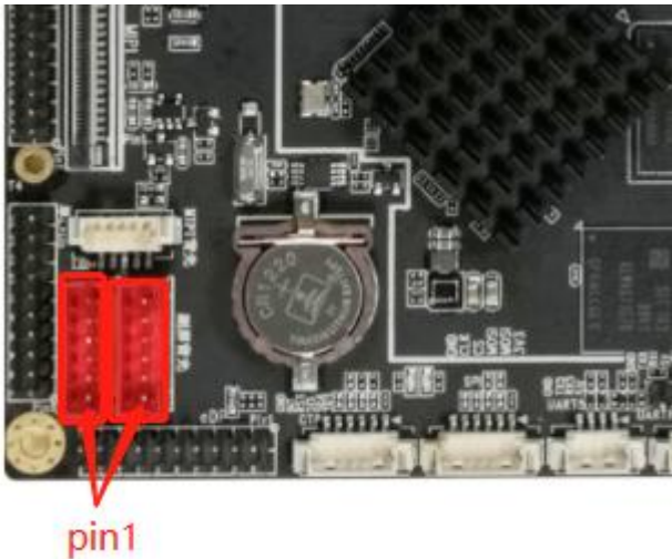
主副屏背光接口
