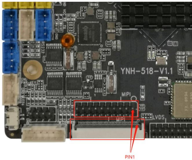
MIPI 接口 (20PIN/2.0mm)
