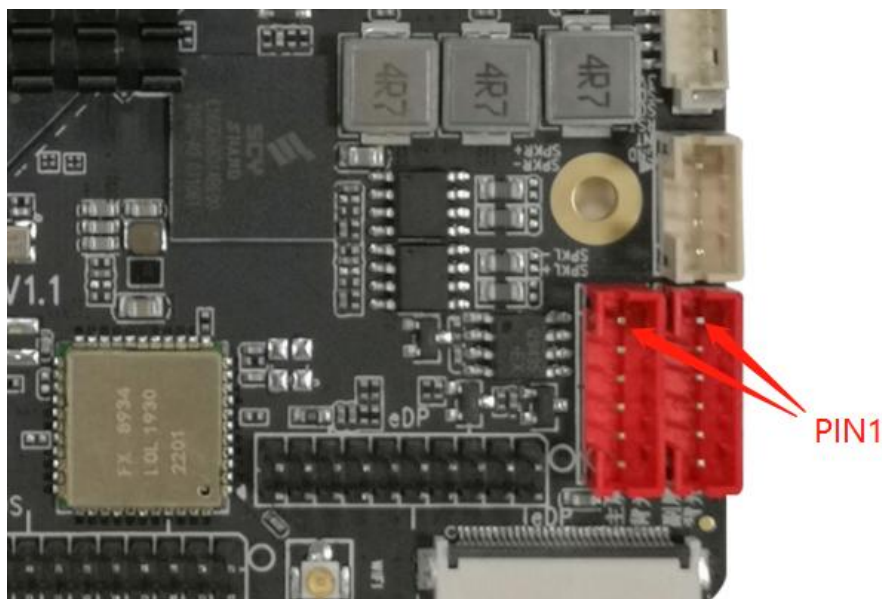
主副屏背光接口
