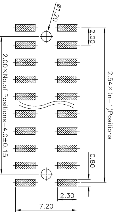
P.C.B LAYOUT
