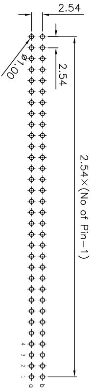
P.C.B LAYOUT
