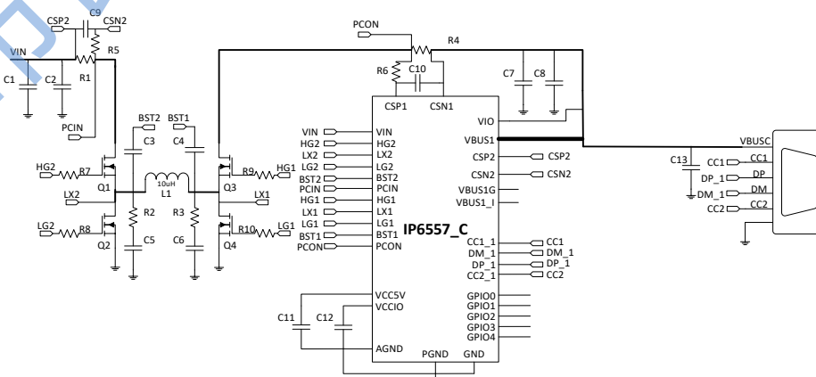
图 1 IP6557 单 C 口的简化应用原理图
