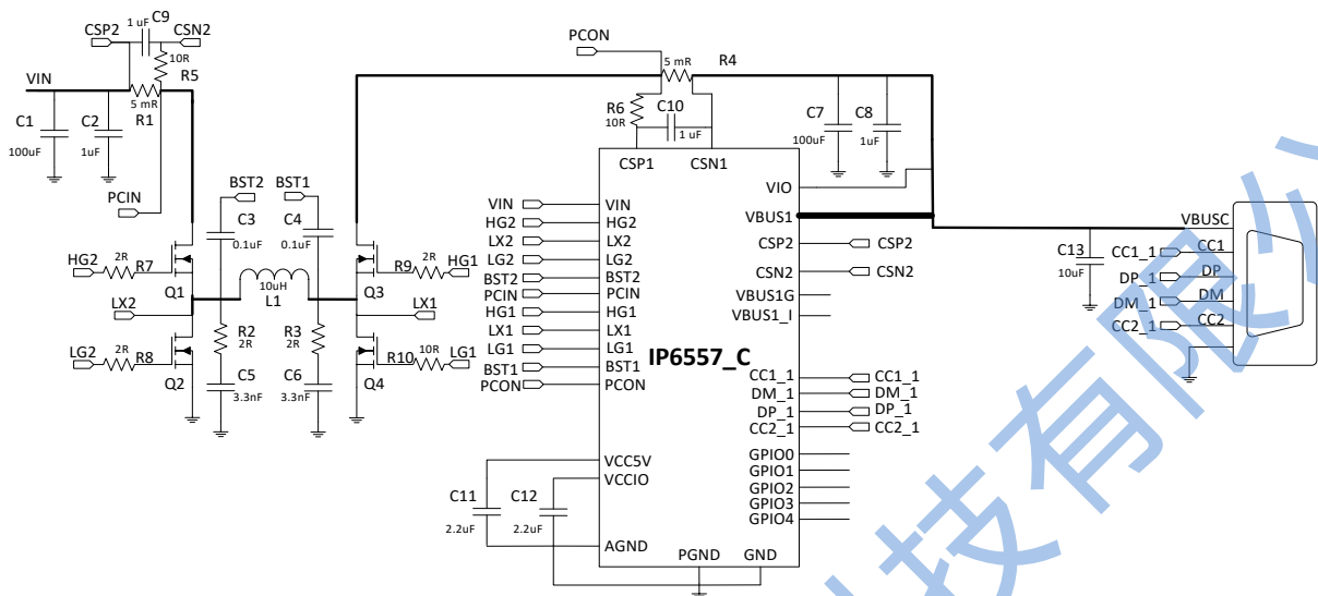
图 9 IP6557 单 C 口的典型应用原理图
