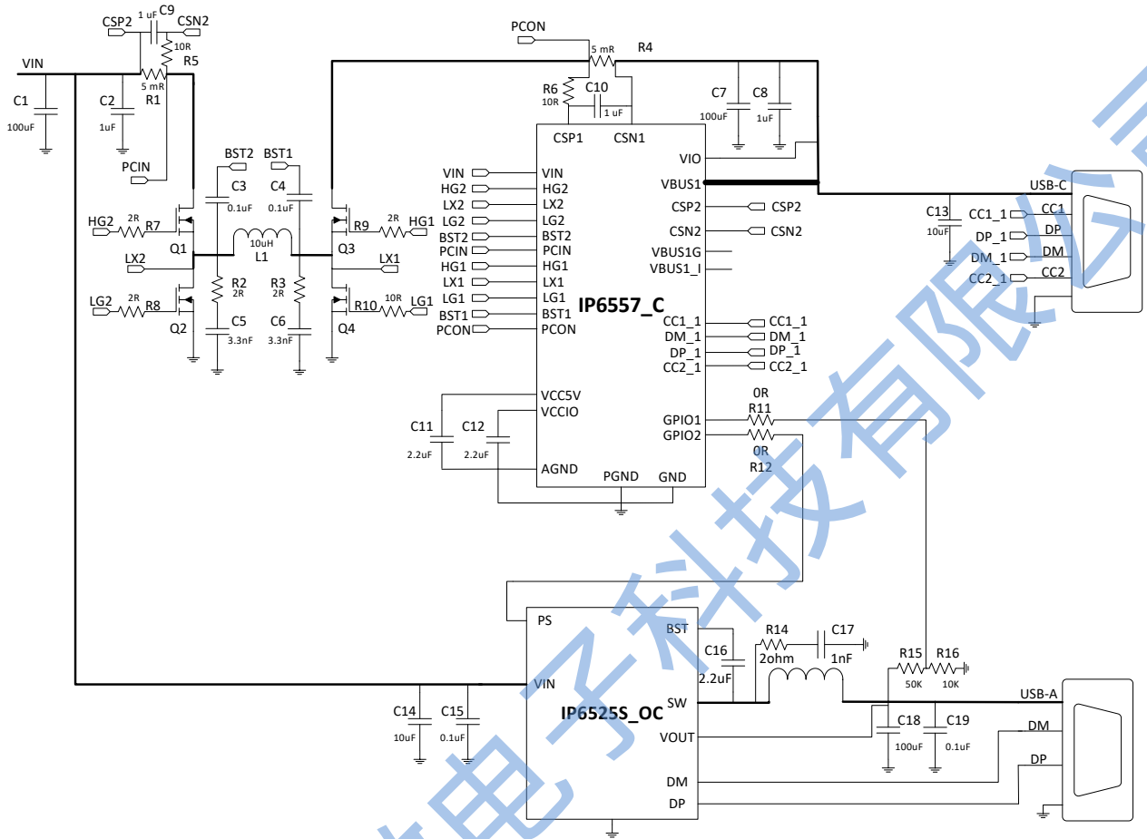
图 11 IP6557+IP6525S_OC 做 USB-A 和 USB-C 双口智能调节输出功率的典型应用原理图
