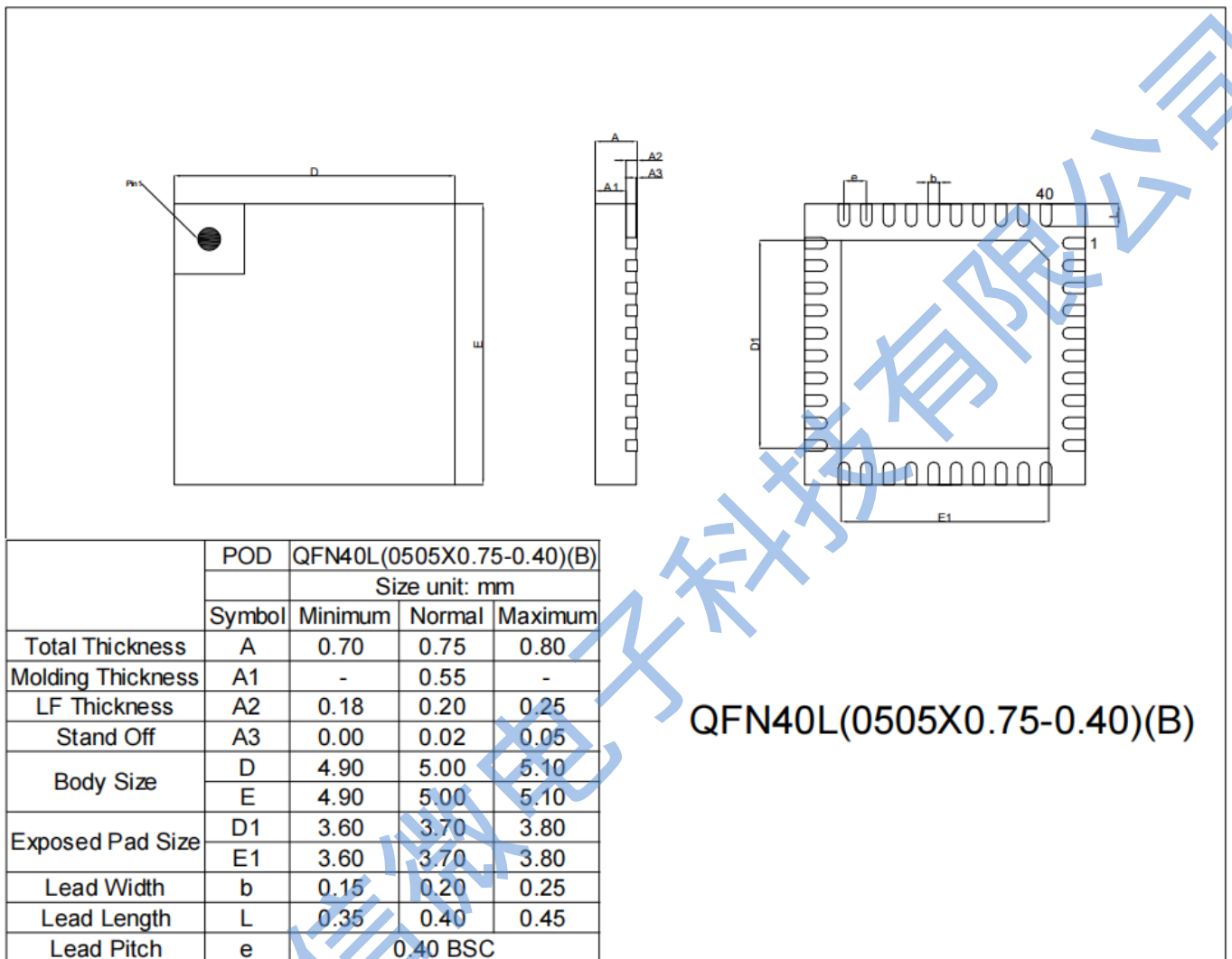
图 12 封装图
