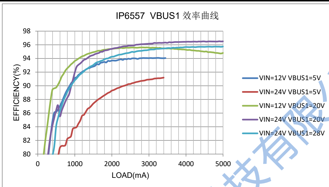
图 5 IP6557 VBUS1 输出效率曲线
