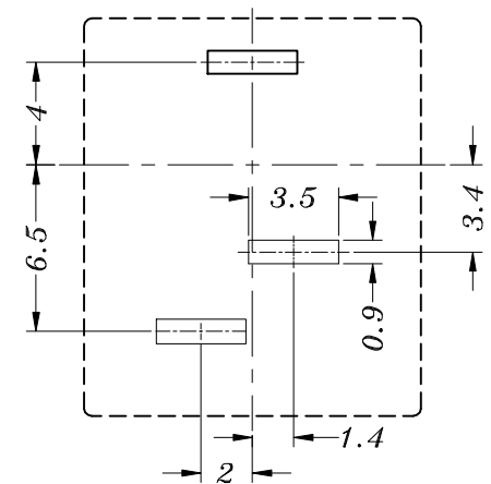
P.C.B LAYOUT
