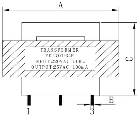
正视图 FRONT VIEW
