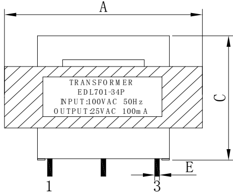
正视图 FRONT VIEW
