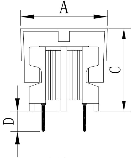
正视图 FRONT VIEW
