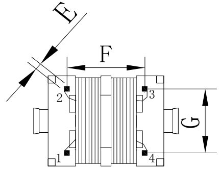
底视图 BOTTOM VIEW
