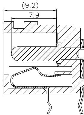
SECTION A-A (插针规格: Ø2.0 & Ø2.5)
