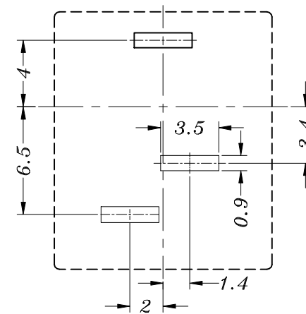
P.C.B LAYOUT
